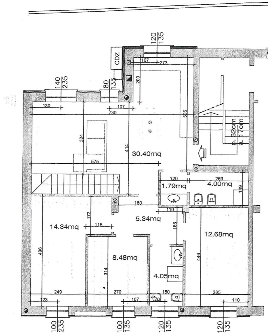
PIANTA PIANO TERRENO
